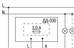
Рисунок 18 – Схема подключения датчика ДД-030
