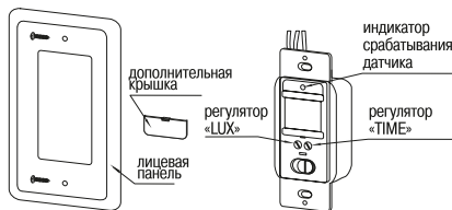
Рисунок 11 – Конструкция датчика движения ДД-028
