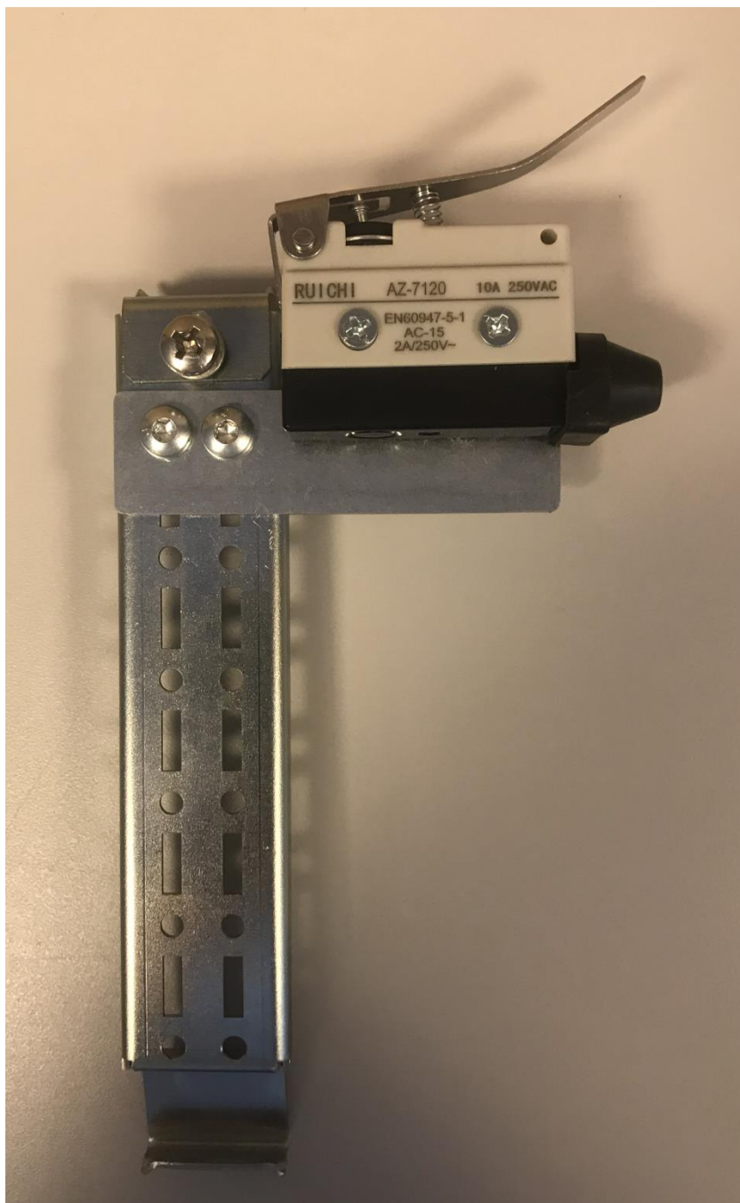
Рис.3.1.8-1 Присоединение монтажной пластины с датчиком вскрытия к шине внутреннего монтажа
