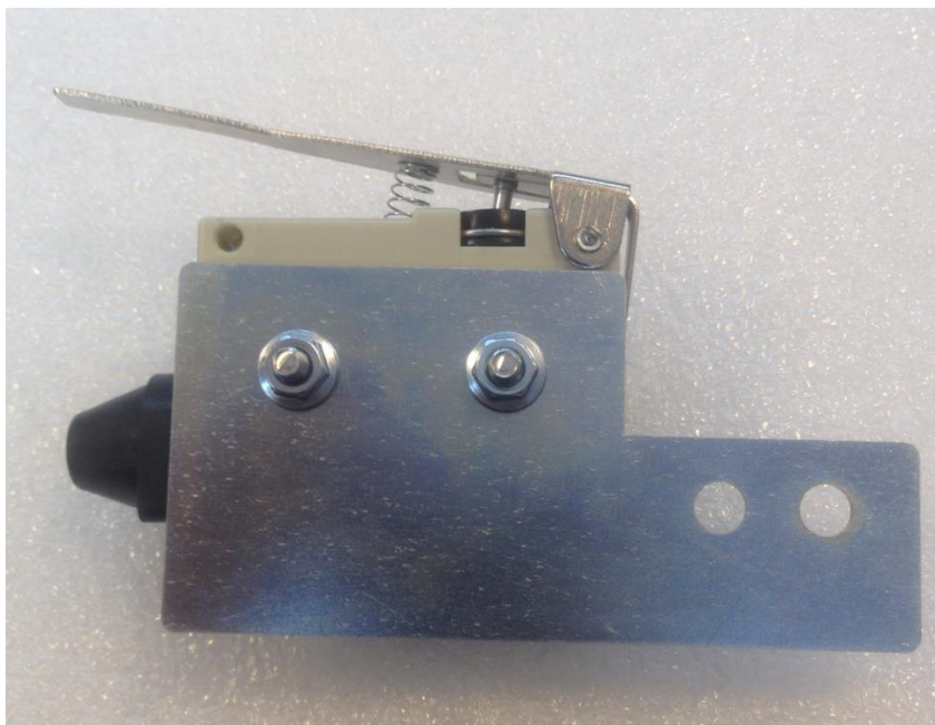
Рис.3.2.7-2 Присоединение датчика вскрытия к монтажной панели
