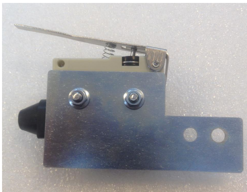
Рис.3.1.7-2 Присоединение датчика вскрытия к монтажной панели
