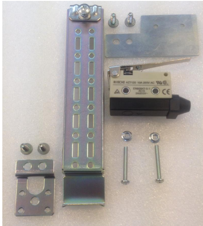
Рис.2.1-1 Комплектация датчик вскрытия для уличных станций
