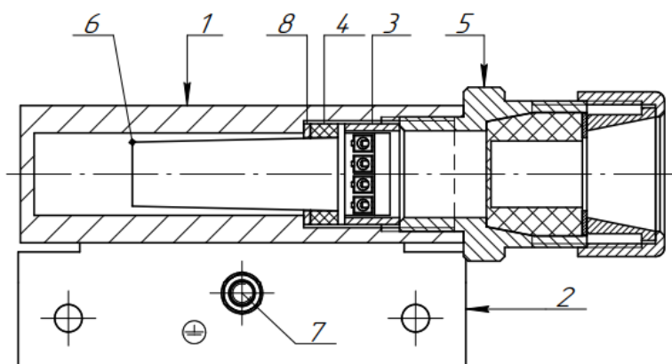
Рис.2 Габаритные и установочные размеры магнитов Ex ДВГ 102
