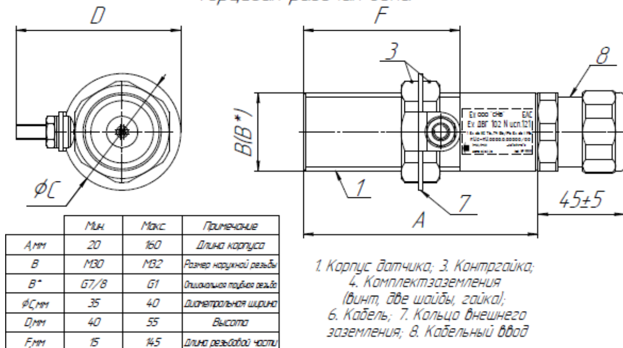
Рис. 1.3 датчик с торцевой рабочей зоной и кабельным вводом
