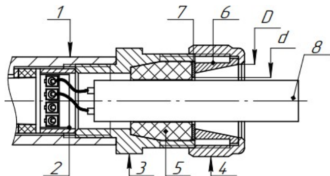
Рис.3 Конструкция и обеспечение взрывозащиты датчика Ex ДВГ 102
