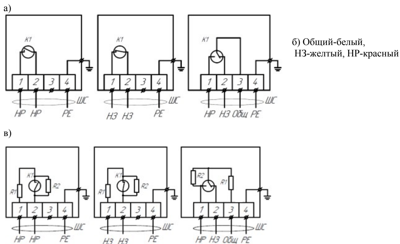
Рис.4 Конструкция и варианты кабельных вводов датчиков Ех ДВГ 102
