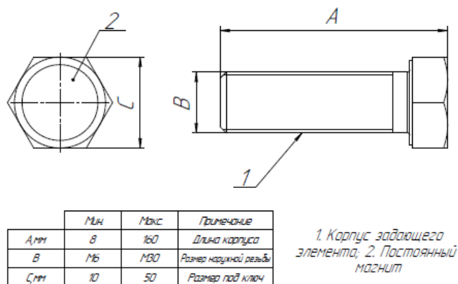
Элемент задающий M220 (221,222,223,224). Торцевая рабочая зона
