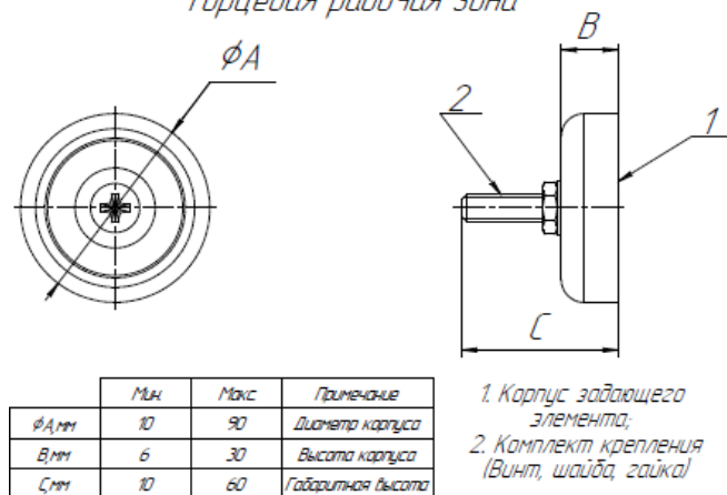
Элемент задающий M210 (211,212,213,214). Торцевая рабочая зона
