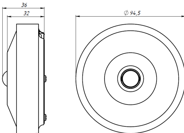
Рис.1 Габаритные размеры датчика.
