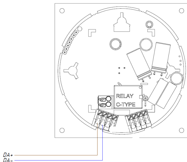
Рис.2 Схема подключения датчика.
