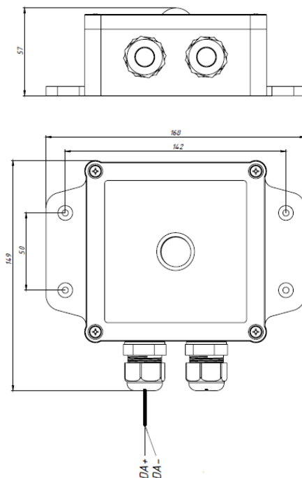
Рис.1 Габаритные размеры и схема подключения датчика
