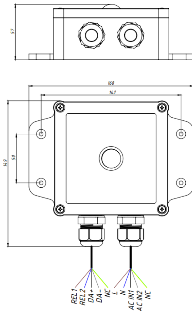
Рис.1 Габаритные размеры и схема подключения датчика
