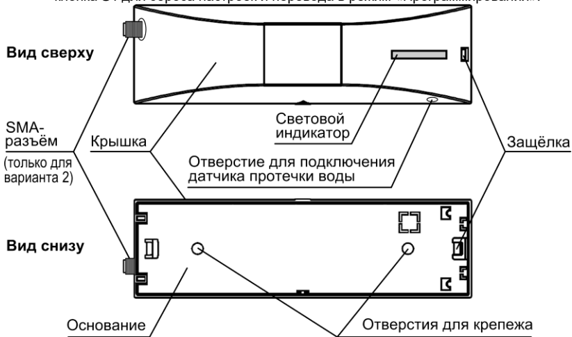
Рис.1 Конструкция сигнализатора. Вид сверху и снизу
