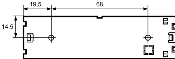
Рис.8 Основание. Присоединительные размеры
