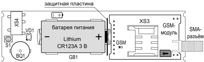
Рис.2 Внешний вид платы контроллера и платы GSM-модуля (SMA-разъём только для варианта 2)
