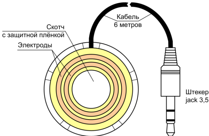
Рис.3 Датчик протечки воды
