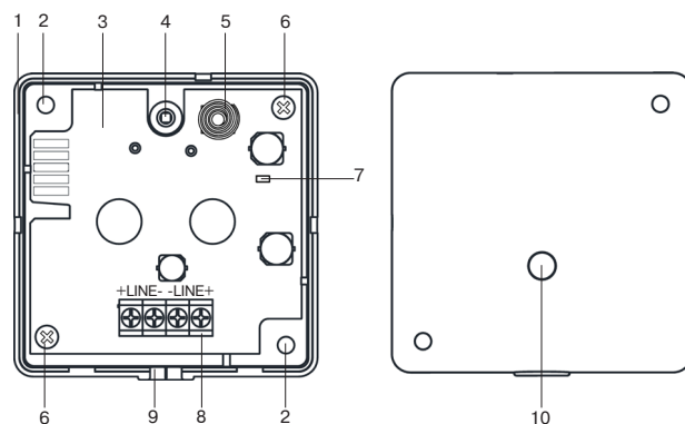
Рисунок 1 – Основание корпуса с печатной платой
