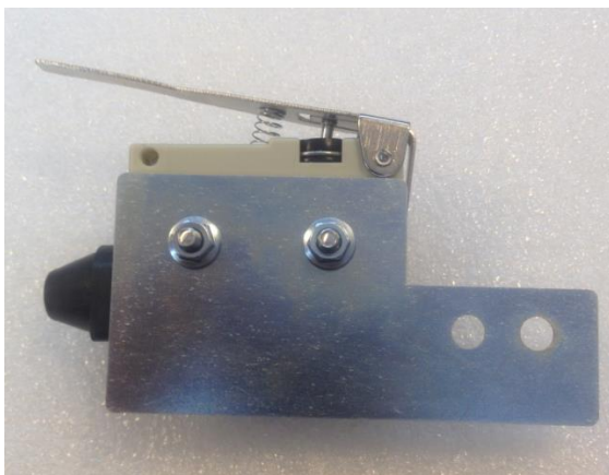
Рис.3.7б Присоединение датчика вскрытия к монтажной панели
