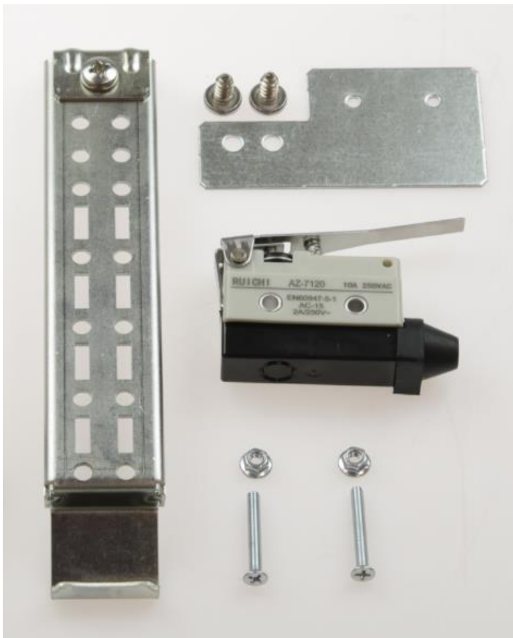
Рис.2 Комплект поставки датчика вскрытия для уличных станций OS (металлический корпус).
