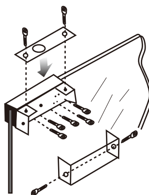
Схема установки
