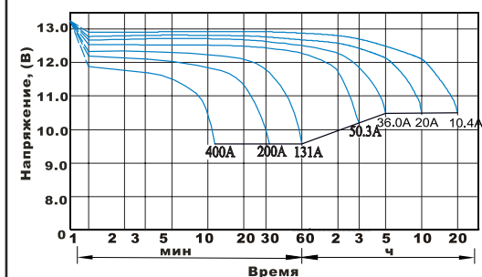
Разрядные характеристики (25°C)
