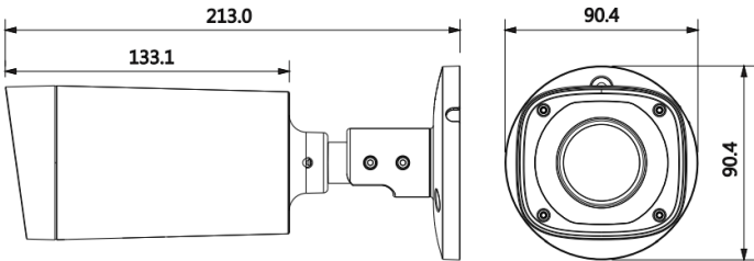
Размеры(мм)
