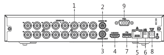
DHI-XVR4116HS-S2
