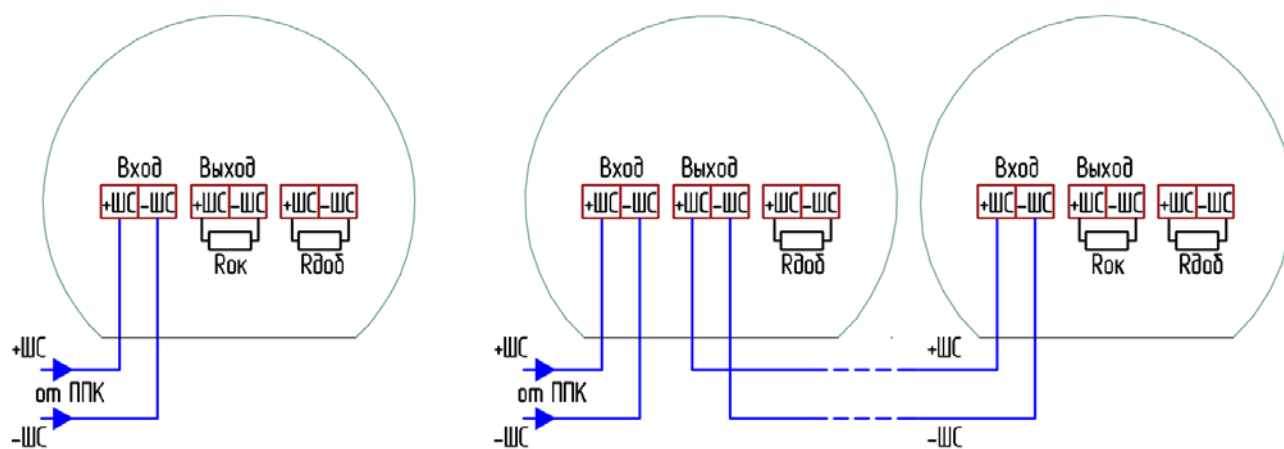
Рисунок Б1. Подключение одного извещателя - слева, нескольких извещателей - справа
