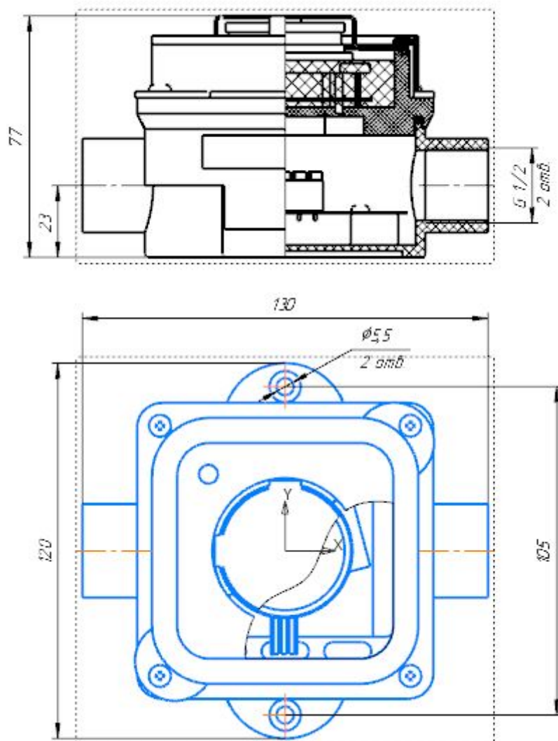
Рисунок А1. Габаритные размеры дымового точечного извещателя Спектрон-ДИП-31-Exi/Exm
