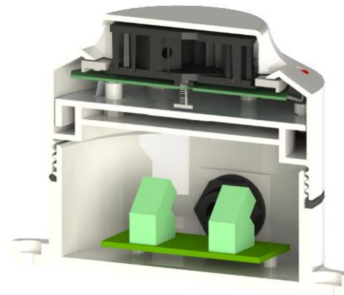
Рисунок 2 – Конструкция извещателей ИП212-44Ex в разрезе
