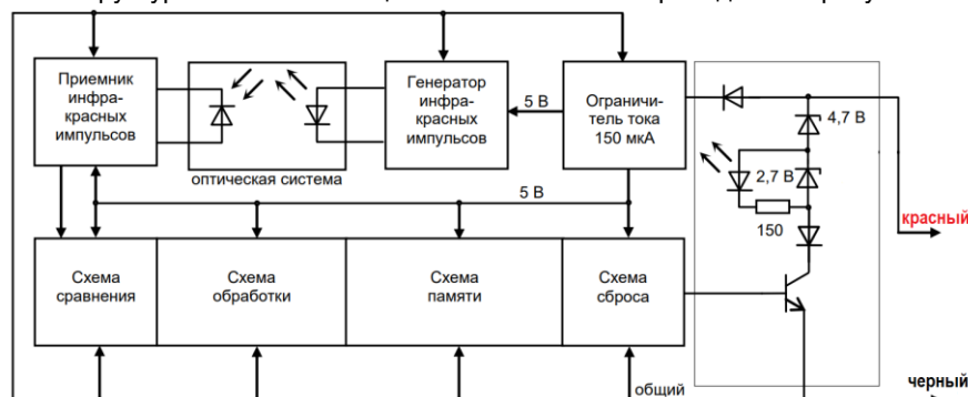
Рисунок 1 – Структурная схема извещателя ИП212-44Ex
