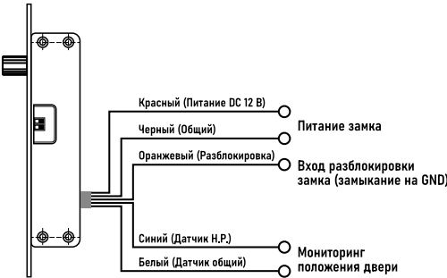
Рис. 5 Подключение замка
