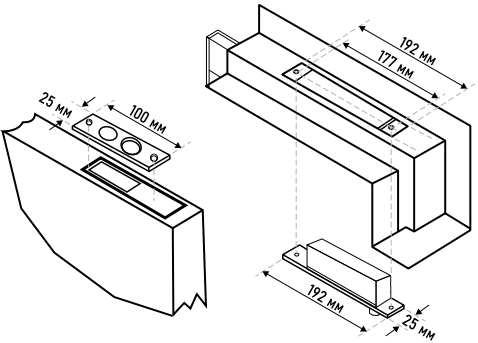
Рис. 4 Установка замка
