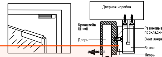
Рис. 4 Монтаж на стеклянную дверь с помощью кронштейна U-типа (УН××0)
