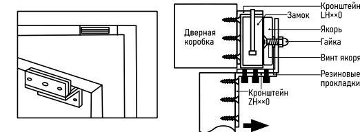
Рис. 3 Монтаж с помощью кронштейна L и Z-типов (ЛН××0, ЗН××0)
