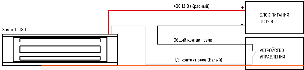
Рис. 9 Схема подключения электромагнитного замка DL180
