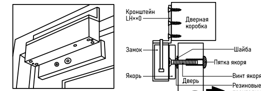
Рис. 2 Монтаж с помощью кронштейна L-типа (ЛН××0)
