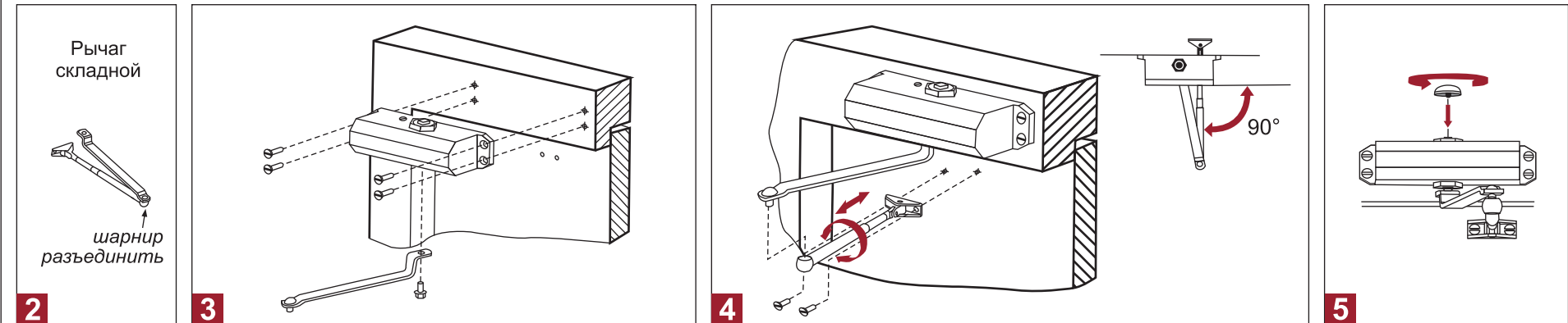
Дверь открывается от себя 90°/120°/180°
