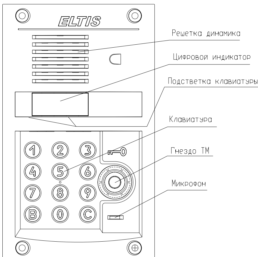
Рис.1 Внешний вид со стороны лицевой панели блока вызова DP303-TD22.
