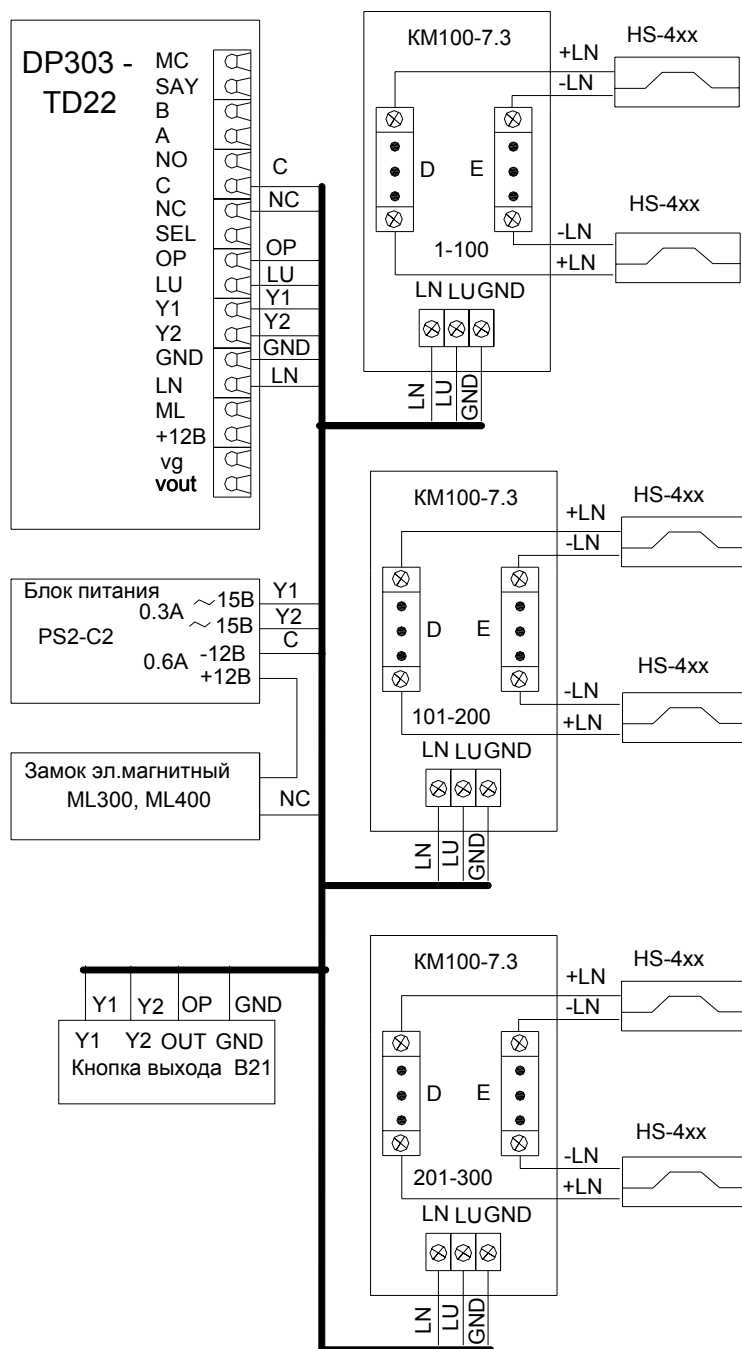
Рис.3 Пример схемы подключения DP303-TD22 в составе домофонного комплекса.
