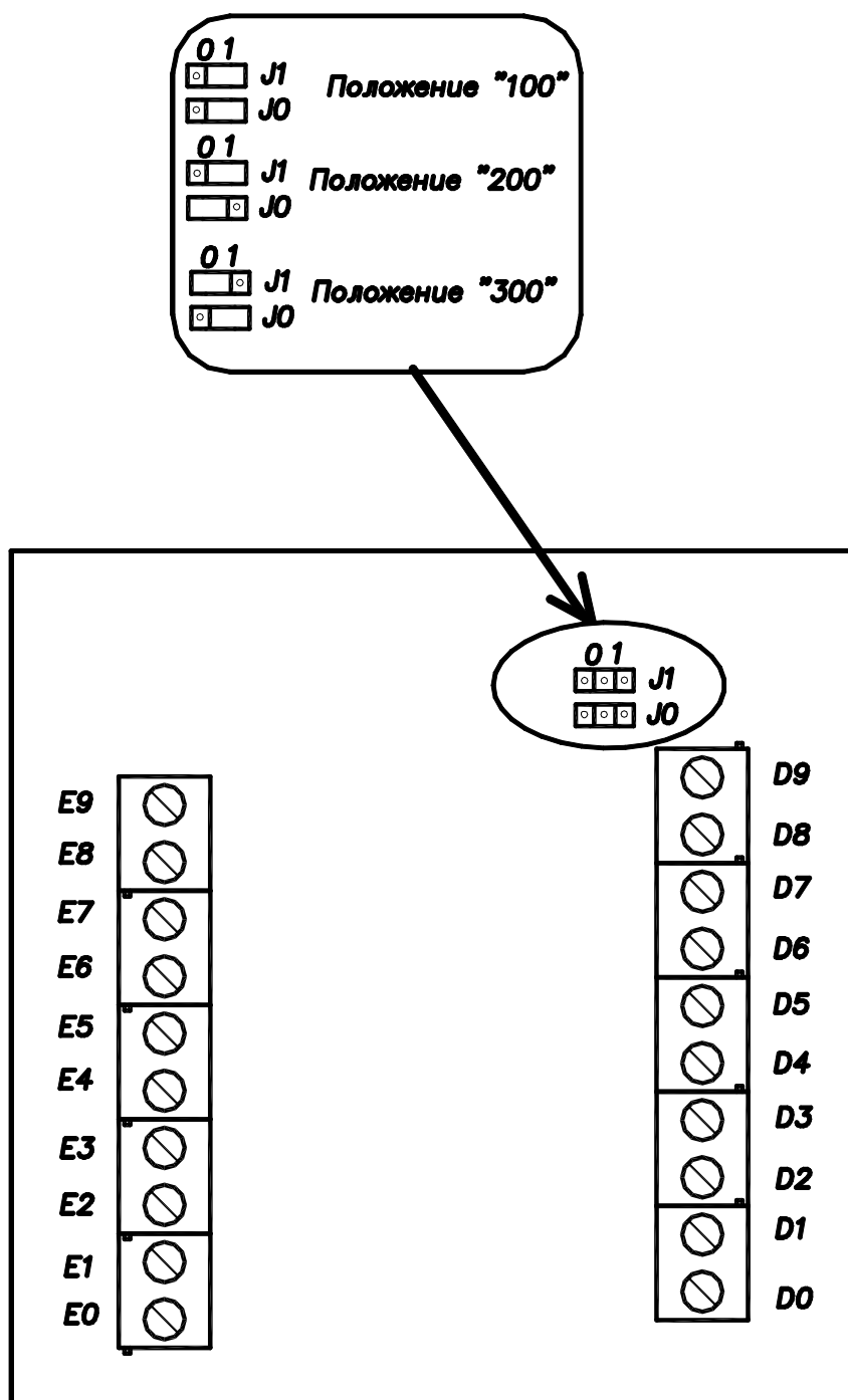
Рис4. Установка джамперов в коммутаторе KM100-7.3
