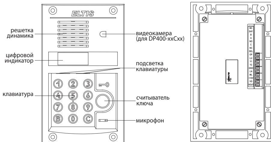
Рис.16 Внешний вид блоков вызова DP400-RD(C)24 и DP400-TD(C)22
