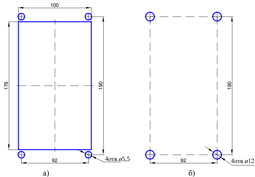
Рис1. Разметка под крепление DP400-TD22 а) снаружи; б) изнутри.
