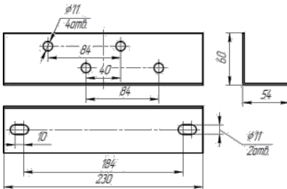
Рис.1 Габаритные и присоединительные размеры кронштейна К-03 АЯКС
