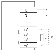
Рис. 1 Схема подключения блока питания мощностью 15-60 ватт.
