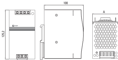
Рис. 4 Габаритные размеры блока питания DR-75W-12, DR-120W-12.
