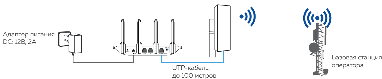
Рисунок 2 - Рекомендуемый способ установки комплекта
