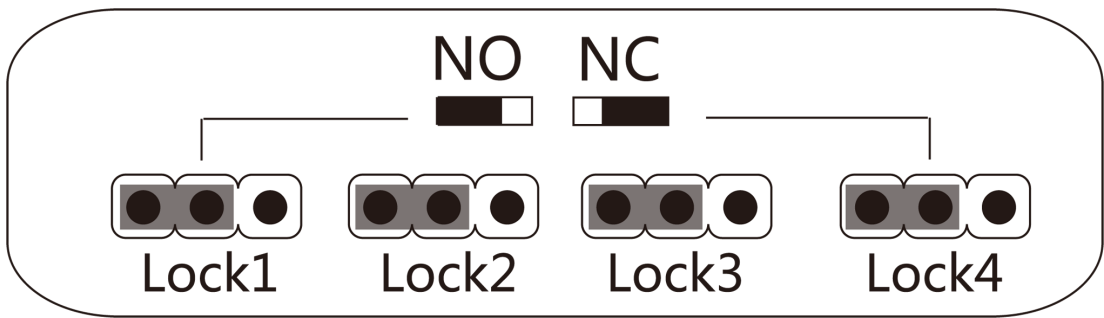
Рисунок 6-3. Состояние NO
