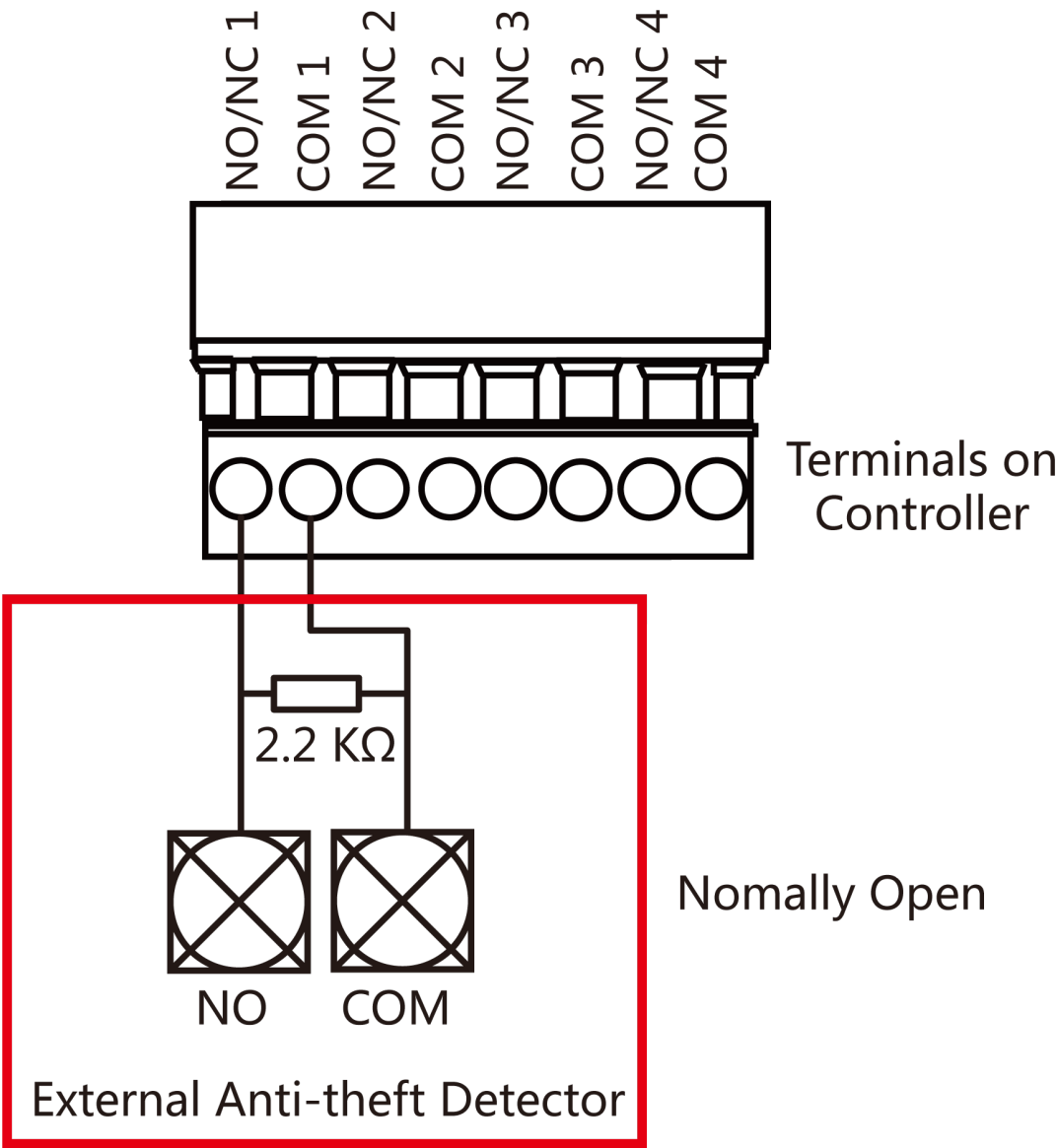
Рисунок 5-12. Подключение NO
