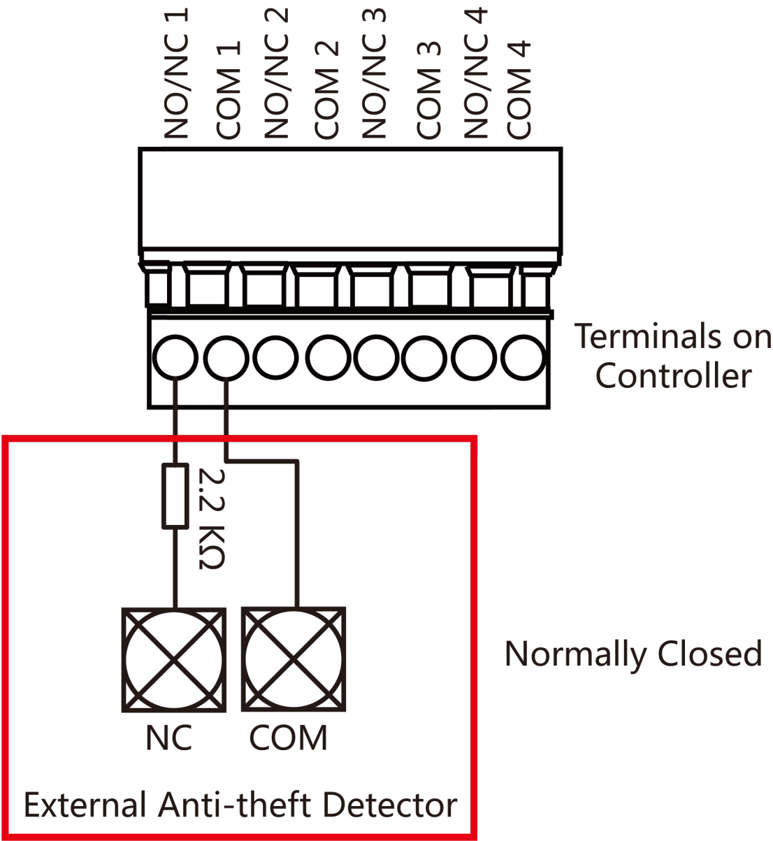
Рисунок 5-13. Подключение NC
