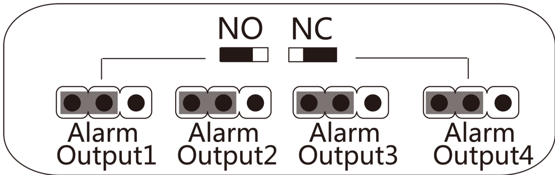
Рисунок 6-5. Состояние NO
