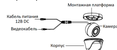
Рисунок 1-15 Камера «шар» I типа Поворот [0° — 360°]
