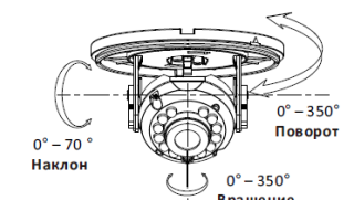
Рисунок 1-12 Настройка угла наблюдения камеры
