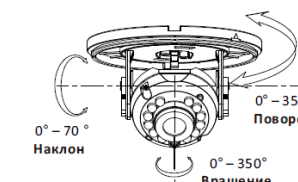
Рисунок 1-12 Настройка угла наблюдения камеры
