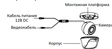
Рисунок 1-15 Камера «шар» I типа Поворот [0° — 360°]
