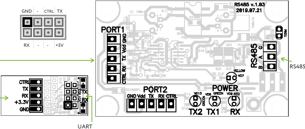
Рисунок 5.2 - Плата RS485
