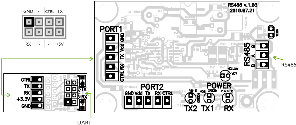
Рисунок 5.2 - Плата RS485
