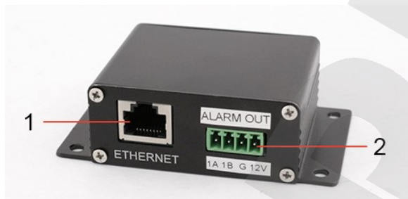
Рис. 3.5. Контроллер NC103 / NC103P
