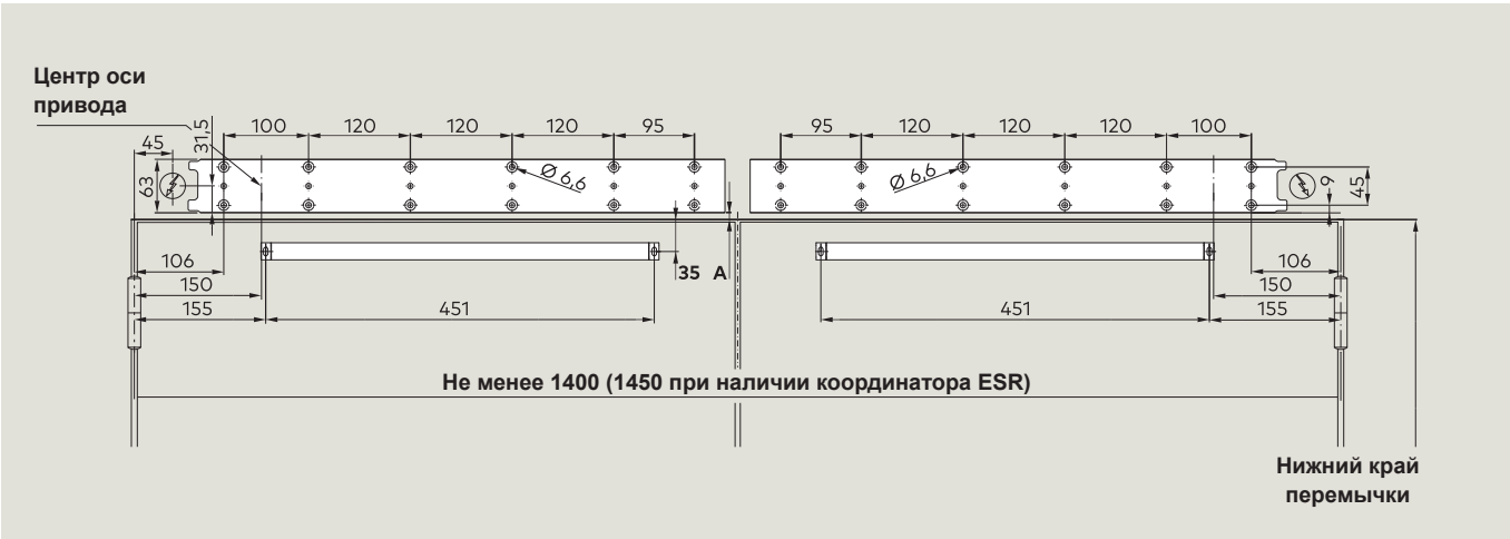
Шаблон для сверления: короткая поворотная ось 12,5 мм
