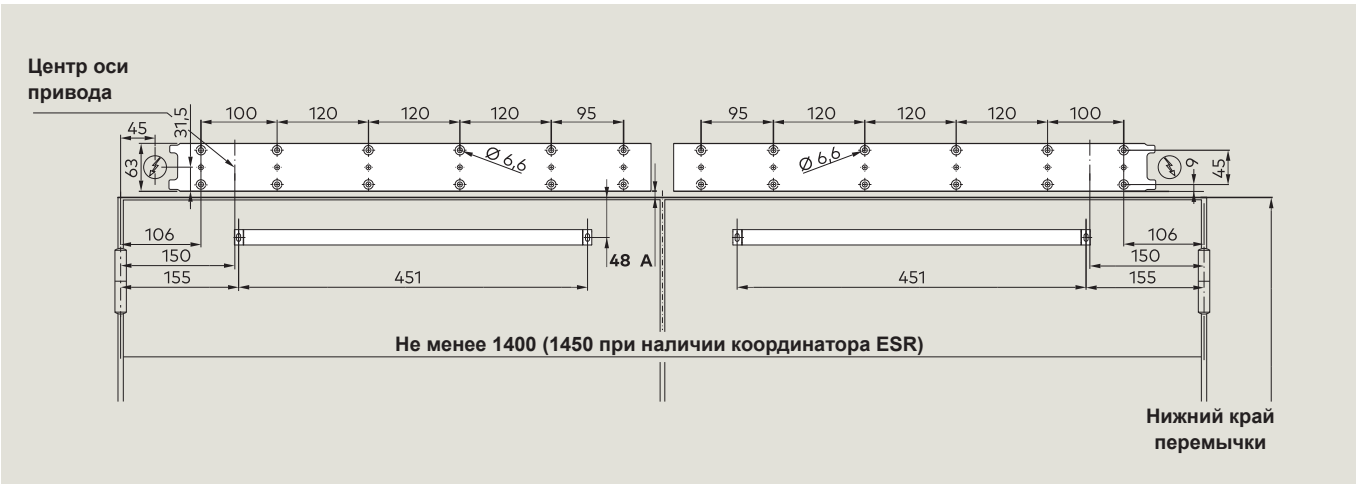
Шаблон для сверления: длинная поворотная ось 25 мм
