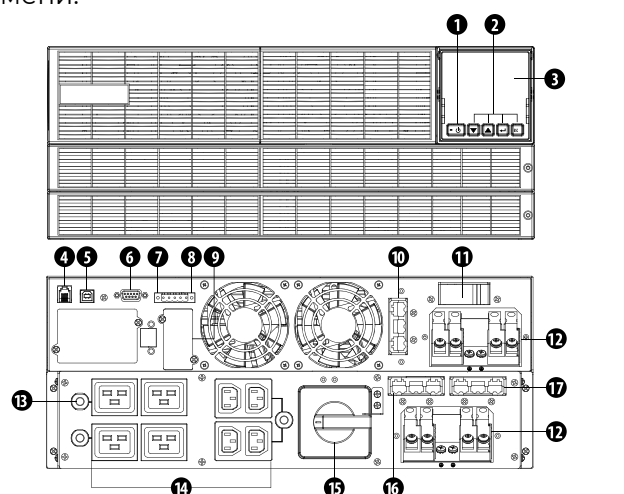
ЭКСПЕРТ-II-6000P, ЭКСПЕРТ-II-10000P
