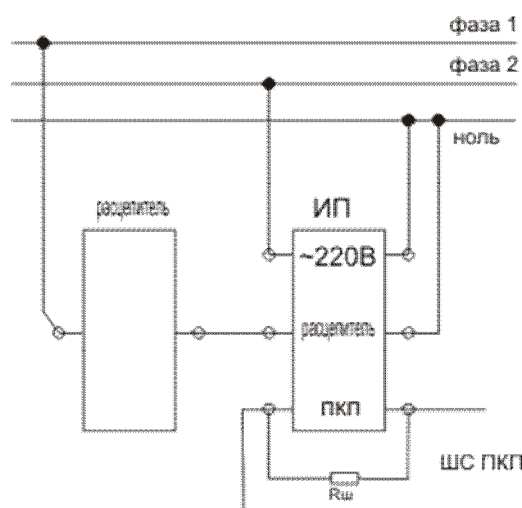
Рис.А.2. – Типовая схема подключения извещателя ИП101/435-3-Р «Эксперт Щит» к ПКП и к распределителю РН-47 при питании от одной фазы, а защите через распределитель – другой. При отключении питания распределителем ИП сохранит питание от другой фазы.
