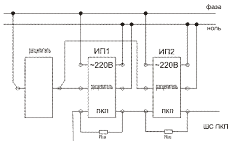
Рис.А.3. – Типовая схема подключения извещателей ИП101/435-3-Р «Эксперт Щит» к ПКП и к распределителю РН-47 с подтверждением выходного сигнала по схеме «И». При отключении питания распределителем ИП1 и ИП2 также обесточатся.
