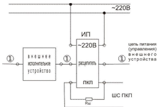
Рис.А.6. – Типовая схема подключения извещателя ИП101/435-3-Р «Эксперт Щит» к ПКП и к внешнему устройству. Внешнее устройство запускается при замыкании цепи питания (управления) ① контактами реле «Расцепитель» на 2-5 сек.
