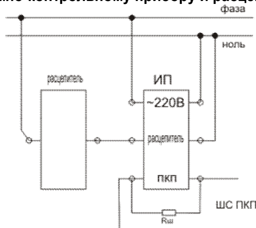
Рис.А.1. – Типовая схема подключения извещателя ИП101/435-3-Р «Эксперт Щит» к ПКП и к распределителю РН-47. При отключении питания распределителем ИП также обесточится.
