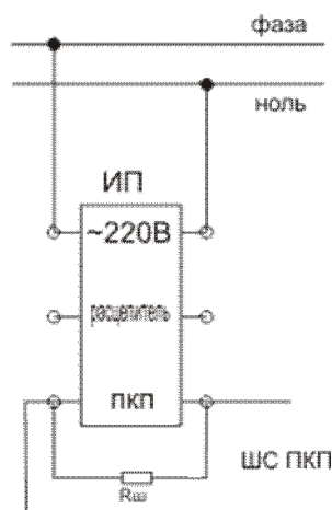
Рис.А.4. – Типовая схема подключения извещателя ИП101/435-3-Р «Эксперт Щит» к ПКП без подключения к расцепителю.
