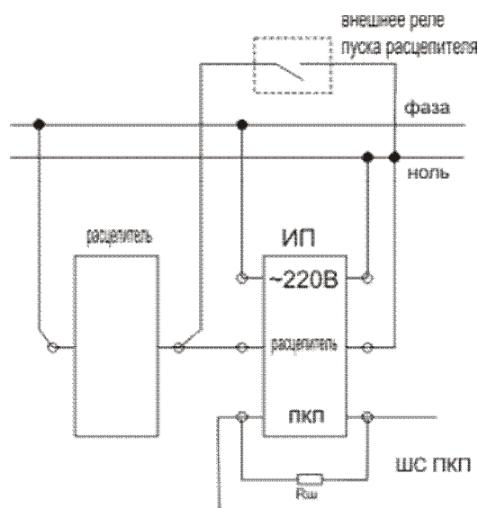
Рис.А.5. – Типовая схема подключения извещателя ИП101/435-3-Р «Эксперт Щит» к ПКП и к расцепителю РН-47. Параллельно контактам «Расцепитель» ИП подключается внешнее реле пуска расцепителя.
