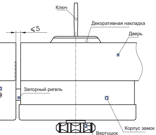
Схема расположения замка и его ответной части
