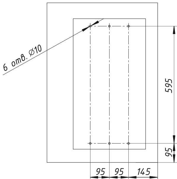
Рис.3 Габариты и разметка крепежных отверстий ключницы RusGuard KeyKeeper - 64
