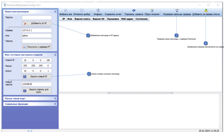
Рис.5 Утилита RusGuardKeyKeeperConfig
