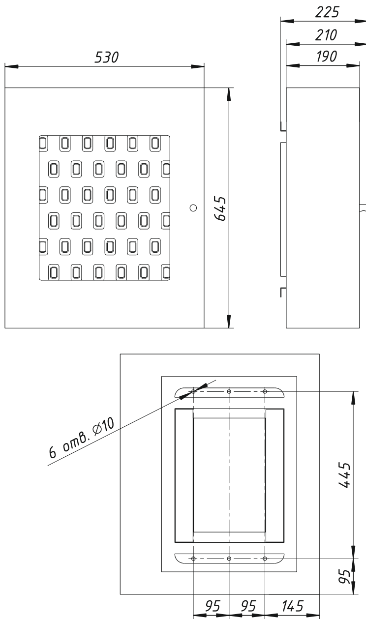
Рис.2 Габариты и разметка крепежных отверстий ключниц RusGuard KeyKeeper - 24, RusGuard KeyKeeper - 48
