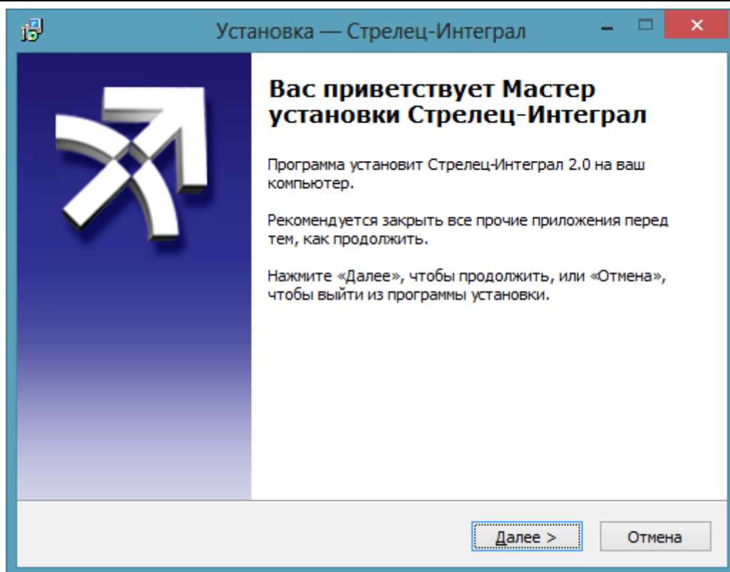
Рисунок 2 – Окно приветствия
