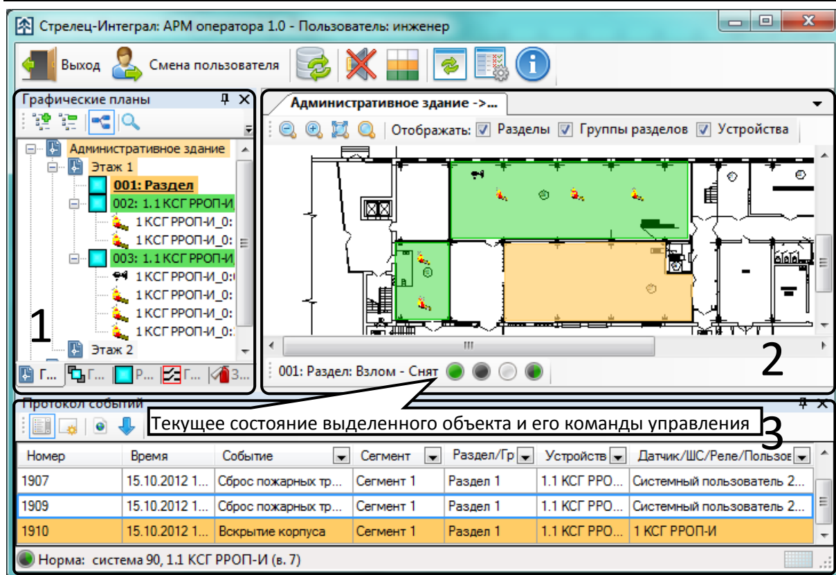
Рисунок 19 – АРМ оператора
