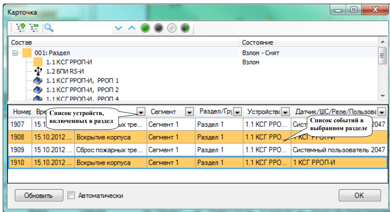
Рисунок 23 – Карточка объекта
