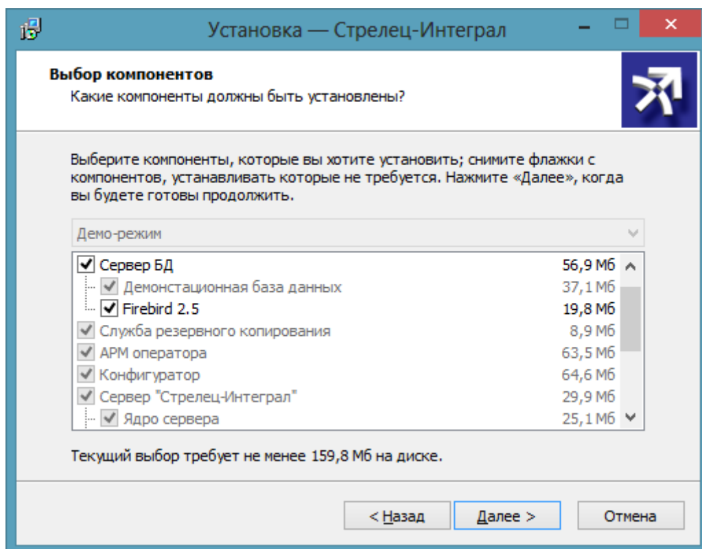
Рисунок 5 – Выбор компонентов
