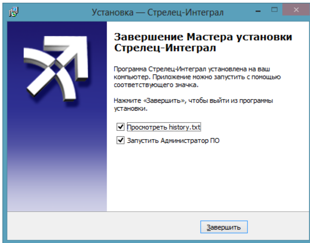
Рисунок 6 – Завершение установки
