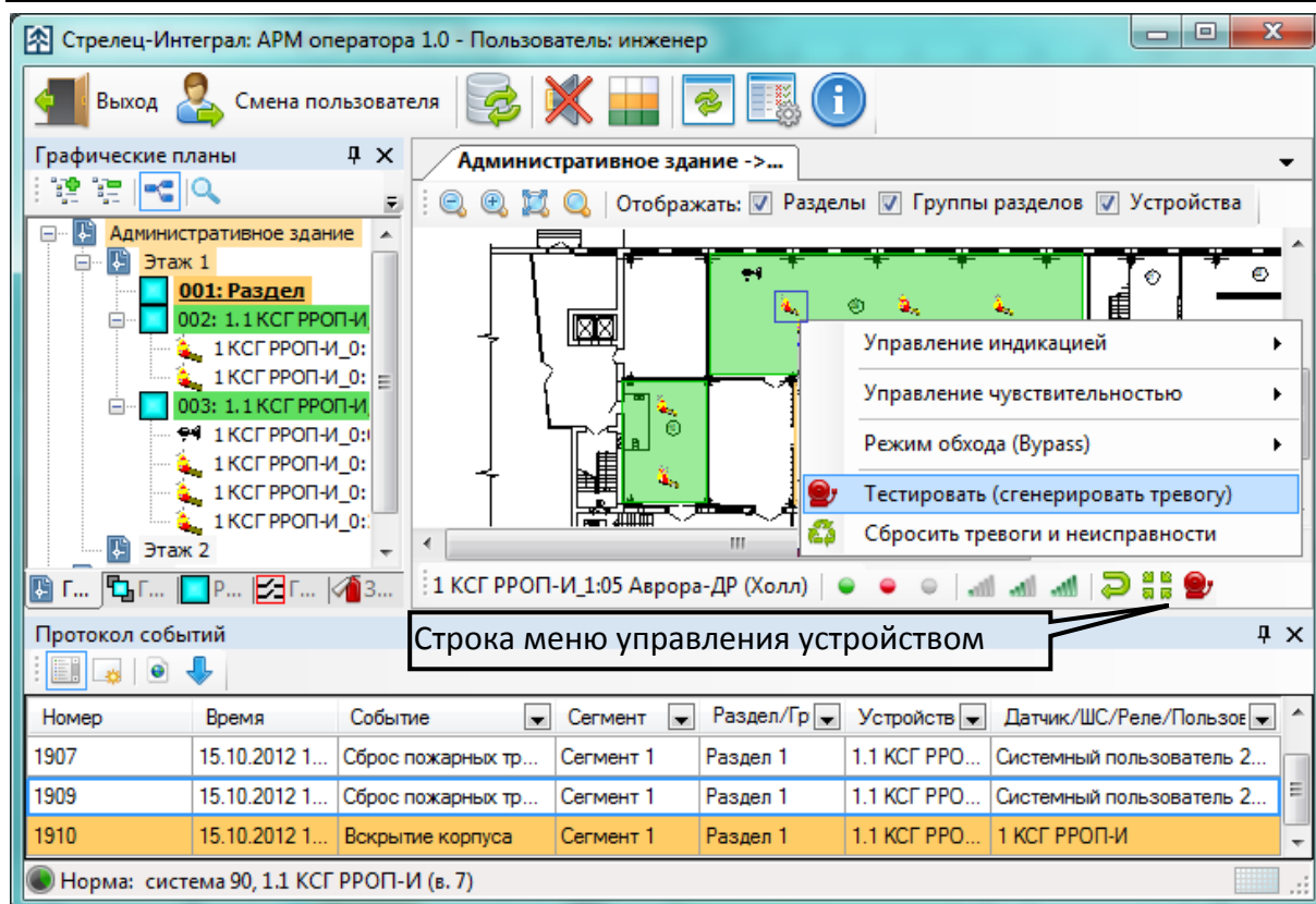
Рисунок 21 – Генерация тревоги
