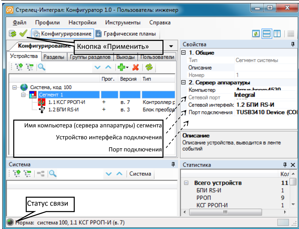
Рисунок 11 – Конфигуратор
