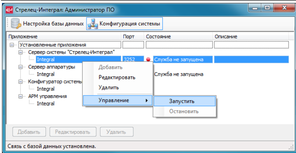
Рисунок 34 – Запуск служб
