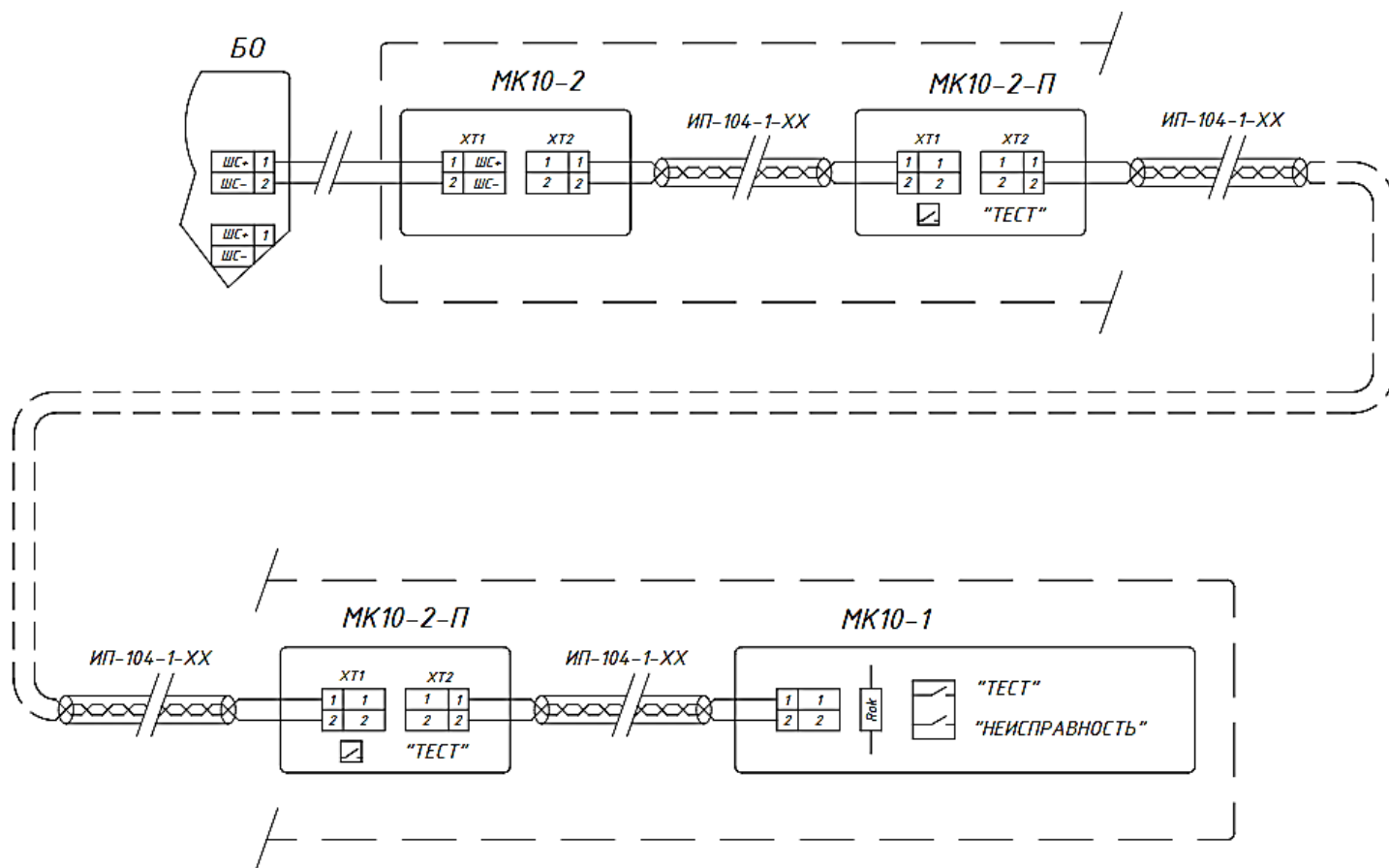
Рис. В3 – Пример использования монтажных комплектов МК10-2-П для срачивания поврежденных участков ЧЭ
