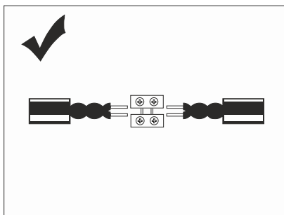
Рис. 9 – Запрещается использовать скрутку для соединения ЧЭ. Следует использовать специальные монтажные комплекты МК10-х, но также допустимо использовать быстрозажимные клеммы или кабельные соединители на винтах с обязательной последующей герметизацией места сращивания.
