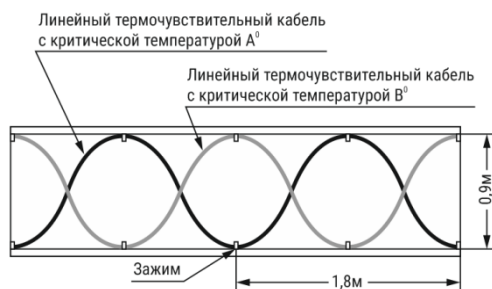
Рис. Д.1 Вариант размещения с двумя ЧЭ в кабельном лотке. Первый кабель выбирается на минимально необходимую температуру, а второй - на шаг больше. Это решение позволяет исключить ложные срабатывания и существенно повысить надёжность раннего обнаружения пожара.
