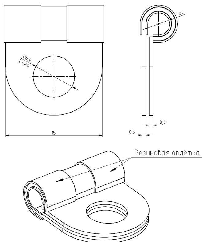
Рисунок Е7. МЭТ-04-02 АЦДР.758579.002 Металлический обрезиненный хомут для крепления термокабеля
