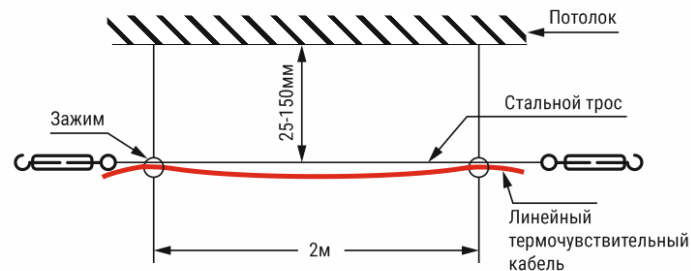
Рис. Д.2 Установка кабеля на потолочных конструкциях. При установке ЧЭ на потолочных конструкциях необходимо соблюдать следующие условия:
