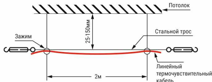
Рис. Д.2 Установка кабеля на потолочных конструкциях.
