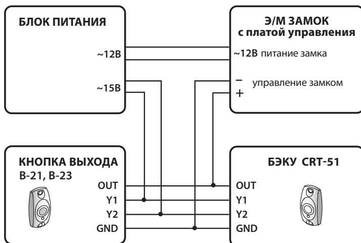
Рис.2 Схема подключения CRT-51 к замку с платой управления и кнопке выхода B-21(B-23)
