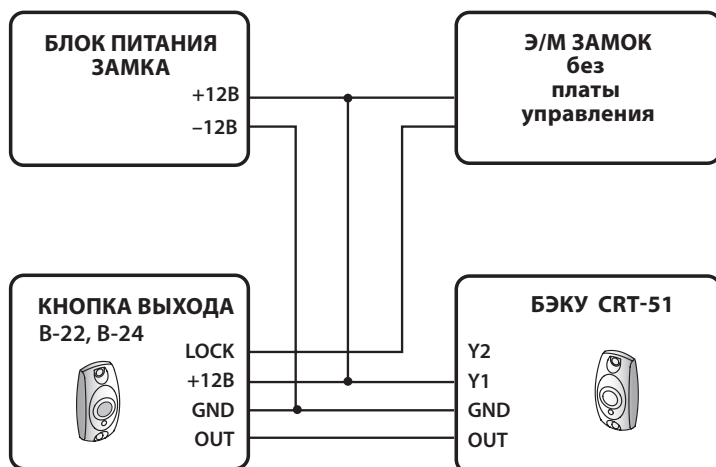
Рис.3 Схема подключения CRT-51 к замку без платы управления и кнопке выхода B-22(B-24)
