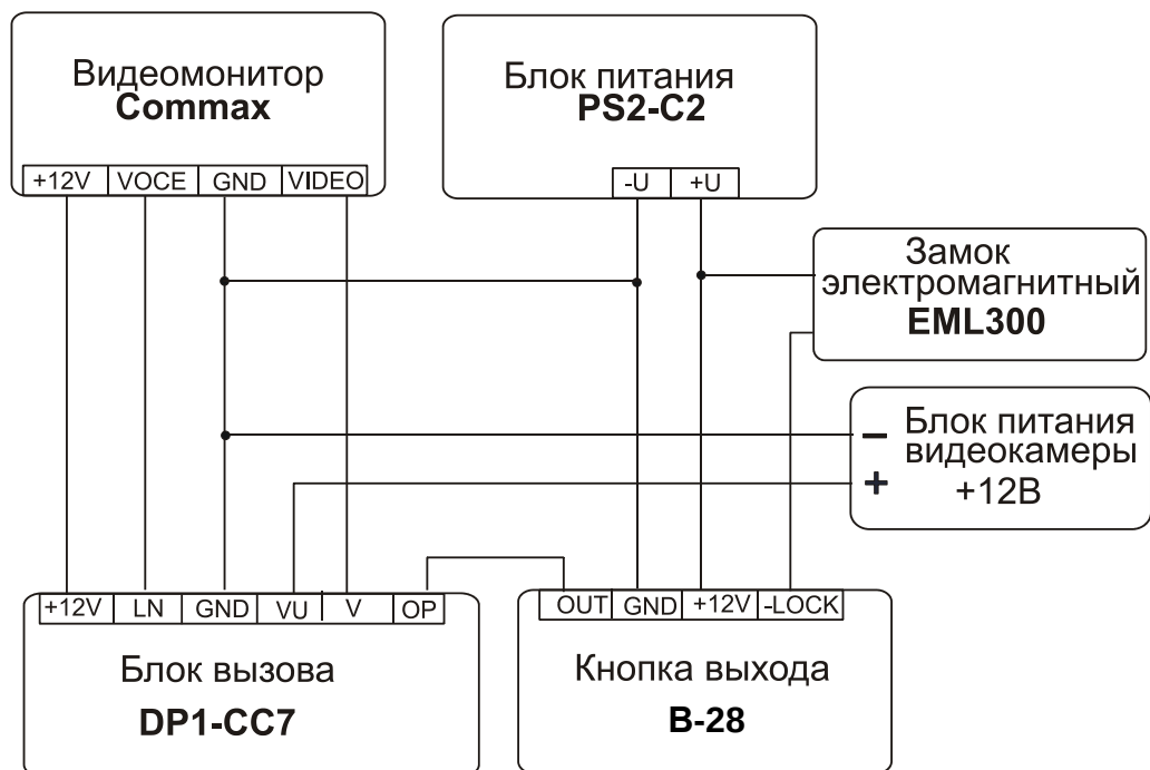
Рис.6 Схема домофонного комплекса с кнопкой вызова B-28
