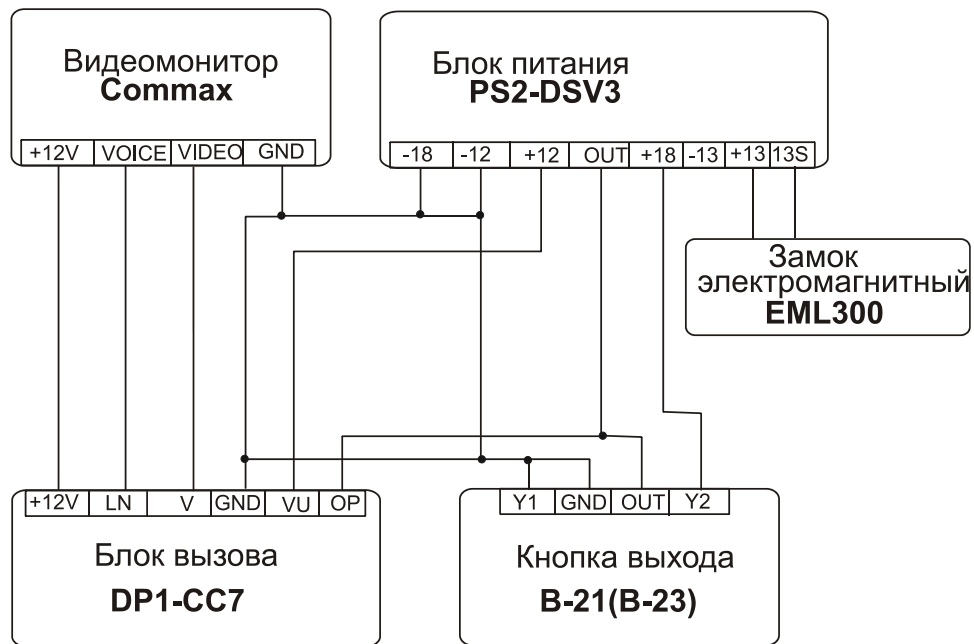
Рис.5 Схема домофонного комплекса с кнопкой выхода B-21(B-23)
