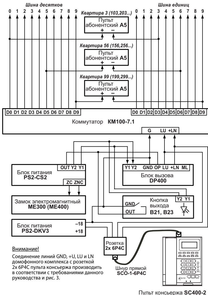
Рис.2 Схема подключения SC400-2 в составе домофонного комплекса
