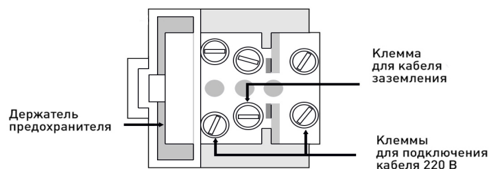
Рисунок 8. Клеммная колодка для кабеля питания
