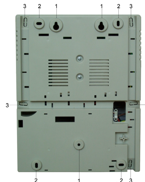
Рисунок 6. Монтажные отверстия
