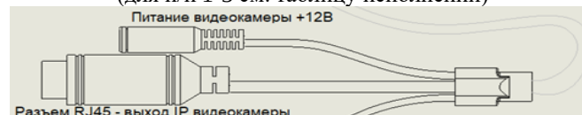
Рис.4 Назначение разъемов видеокамеры EVM2-IPx-M/KP25
