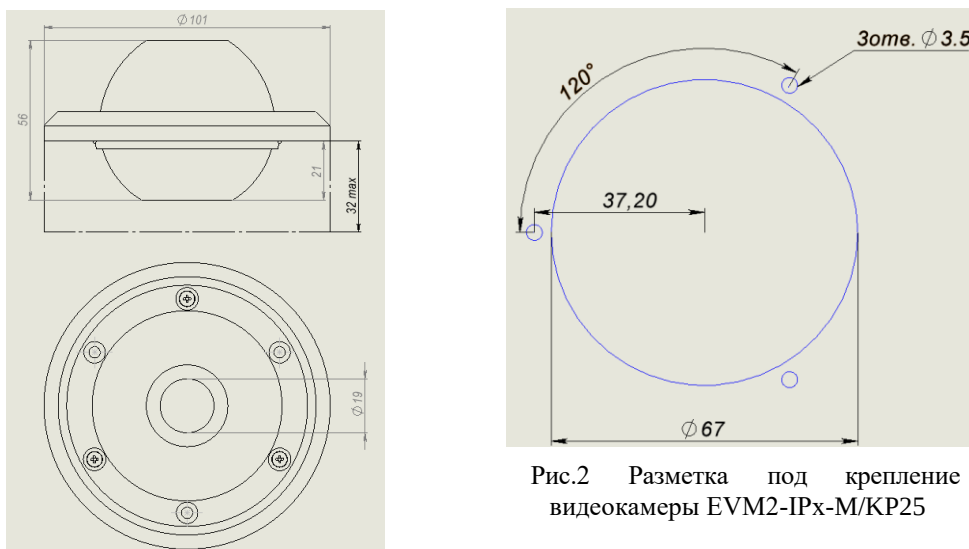
Рис.1 – Внешний вид видеокамеры EVM2-IPx-M/KP25
