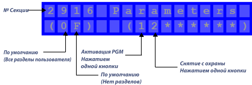
Рисунок 2: Ввод данных для секции [2916] на ЖК-клавиатуре (использовать Список 19 на стр. 38).
