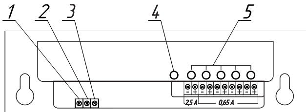
Схема подключения ББП FE-1250 V.5 MAX
