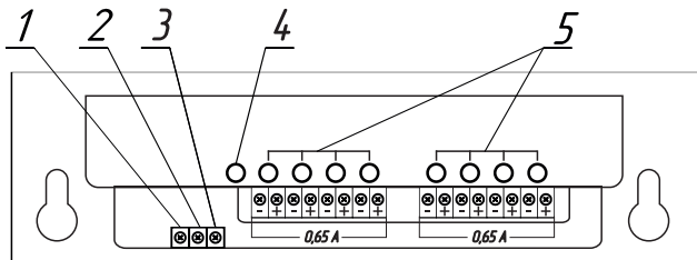
Схема подключения ББП FE-1250 V.8 MAX
