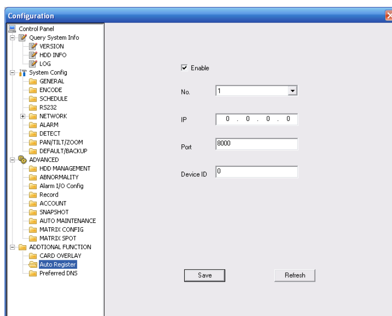
Рис. 7-62 Автоматическая регистрация
