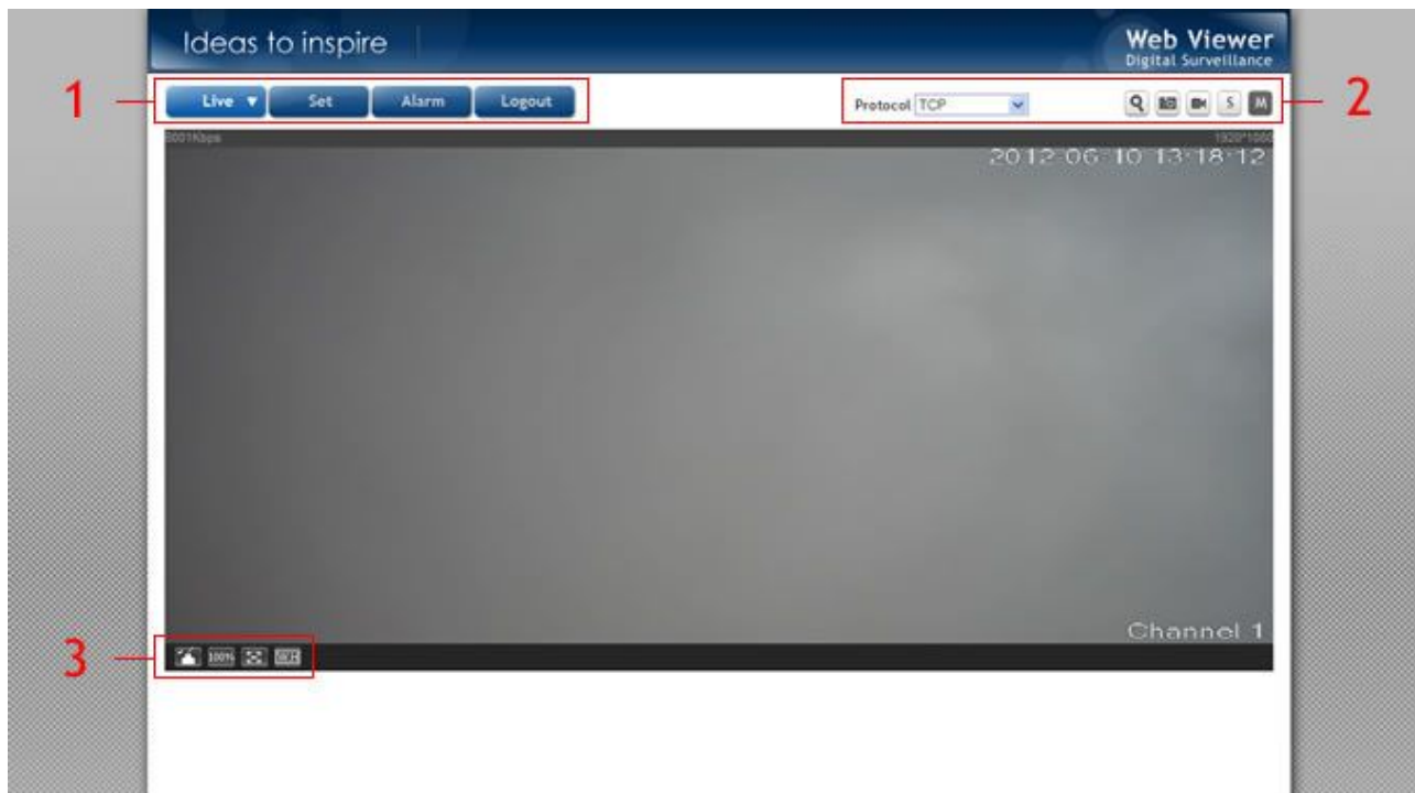
Рис. 2-4 Интерактивный интерфейс
