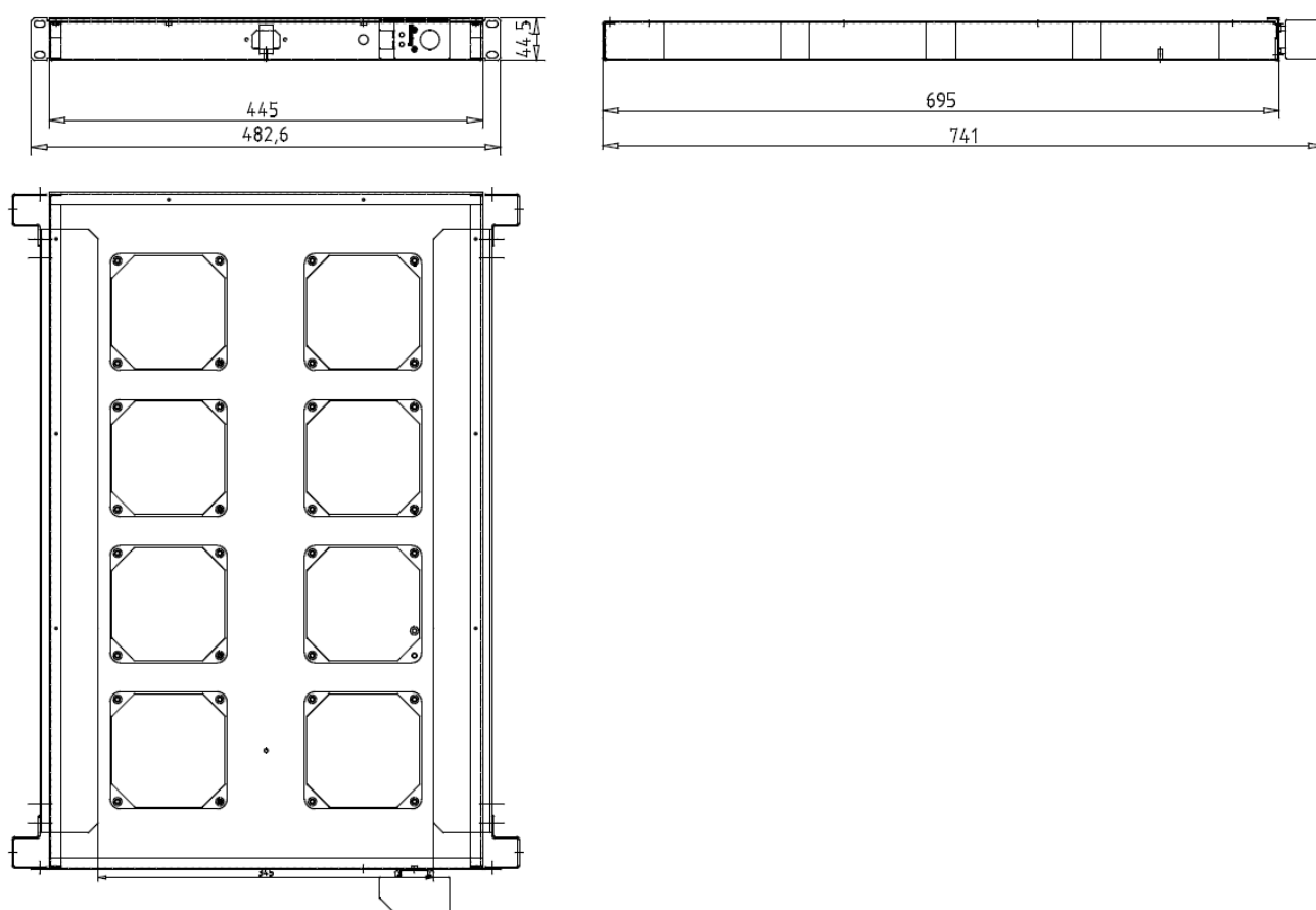
Рисунок 1 – Габаритные размеры изделия
