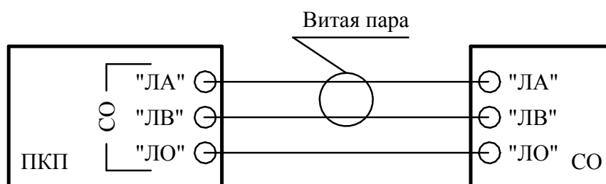
Рисунок 2.4 - Схема подключения настраиваемого СО к изделию
