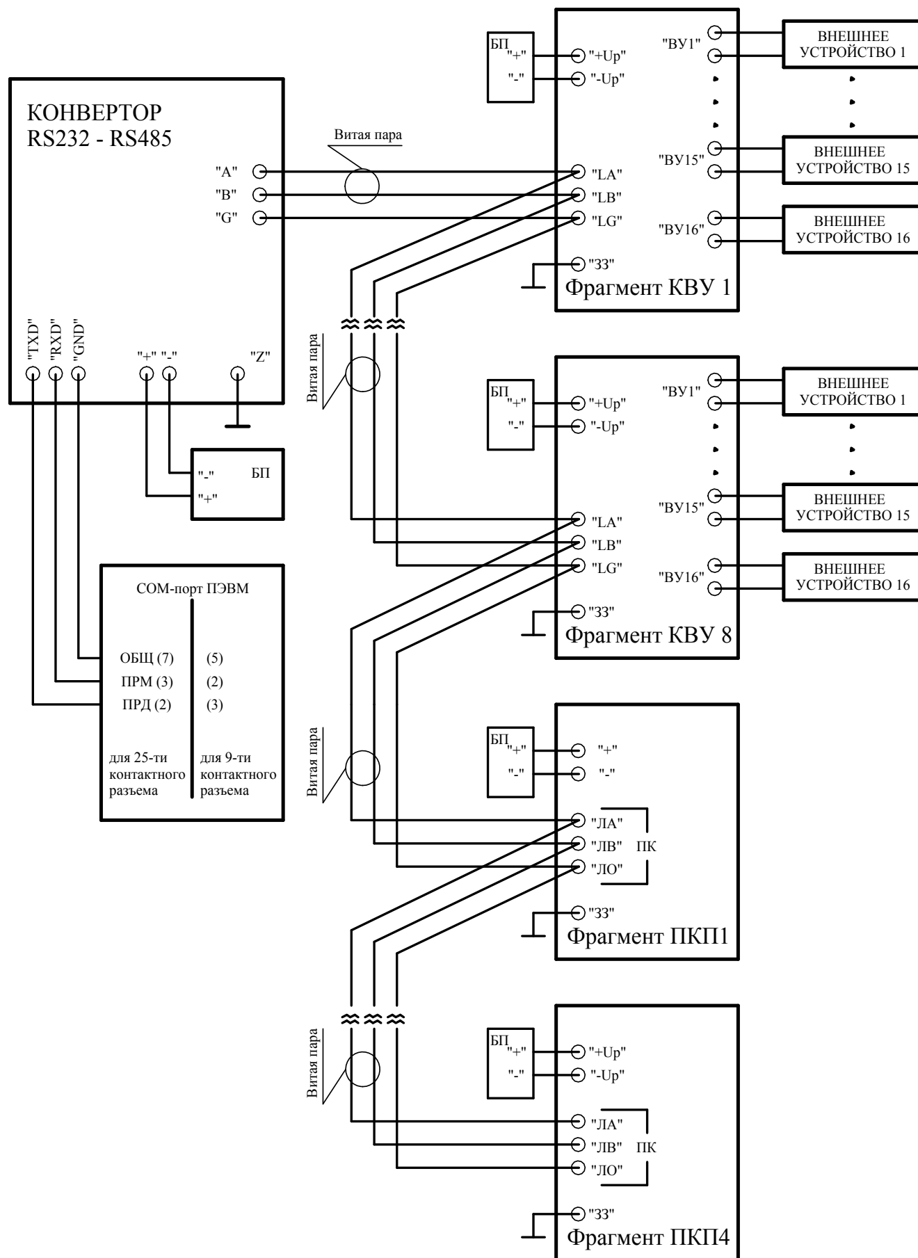
Рисунок 2.5 - Схема подключения изделия, КВУ, конвертора к ПЭВМ
