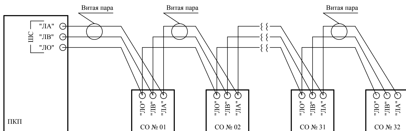
Рисунок 2.3 - Схема подключения контролируемых СО к шлейфу сигнализации изделия
