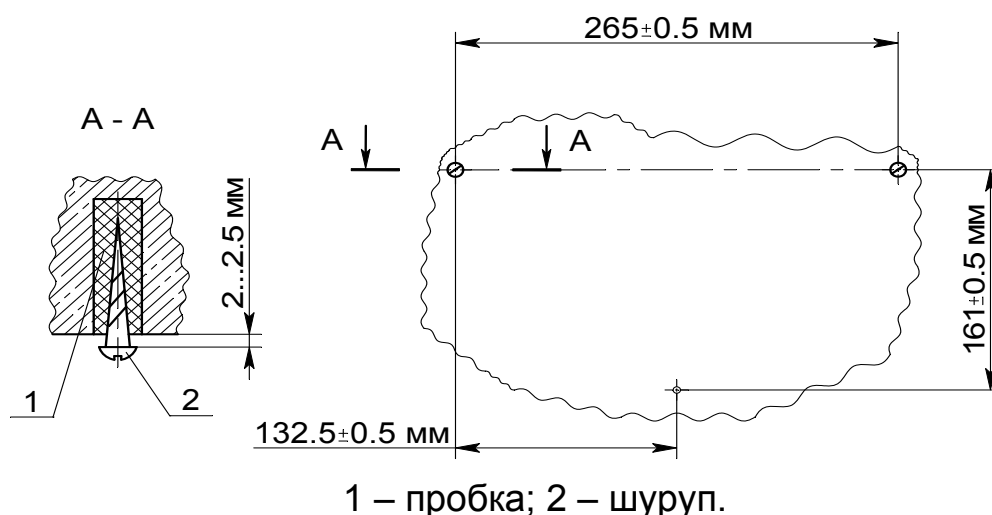
Рисунок 2.1 Разметка для крепление ФОРВАРД32 на вертикальной стене
